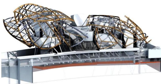
Le centre d'art contemporain de la Fondation Louis Vuitton : la conception architecturale, avec son ossature, ses verrières, son enveloppe opaque dénommée "iceberg" et ses enveloppes vitrées. Le clos couvert du bâtiment est assuré par les façades vitrées et les enveloppes opaque de l'Iceberg, revêtu de Ductal (panneaux en Béton Fibré à Ultra-haute Performance). TESS et © Louis-Marie Dauzat
